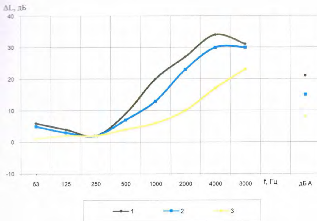
1 – покрытие TecsoundFT75; 2 – покрытие TecsoundFT 55PP; 3 – покрытие SYAl Рисунок 3.1 - Эффективность покрытий на трубе диаметром 200 мм
