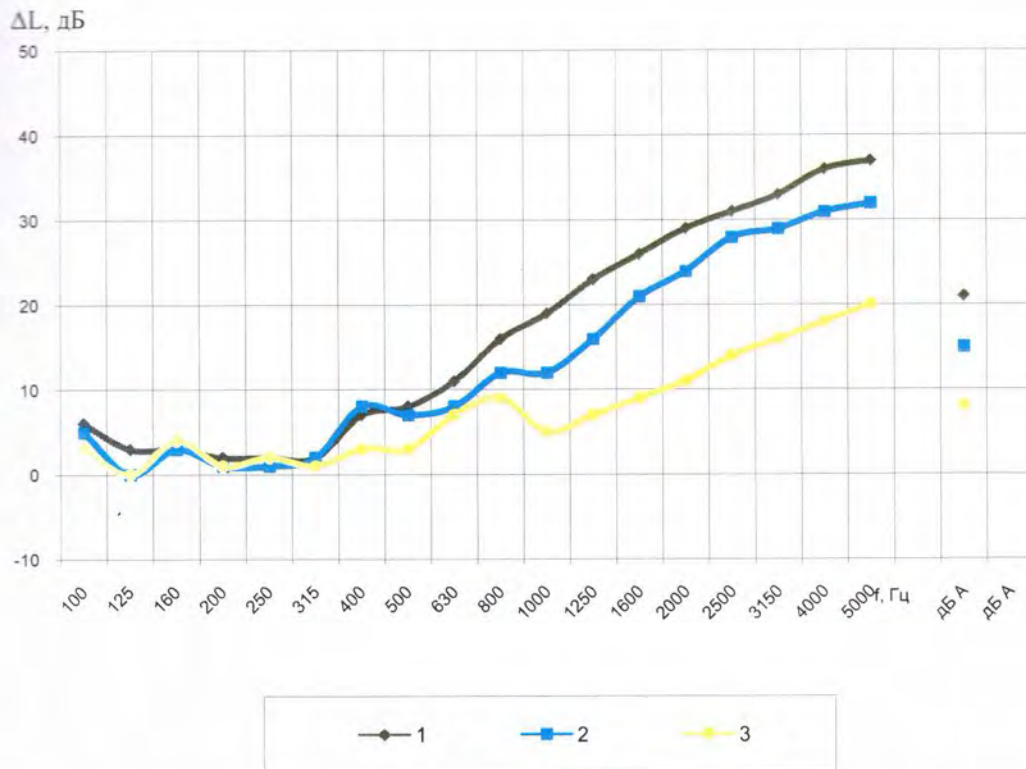
Рисунок 3.3– Эффективность покрытий, установленных на трубу диаметром 200 мм, в нормируемом диапазоне частот звукоизоляции
