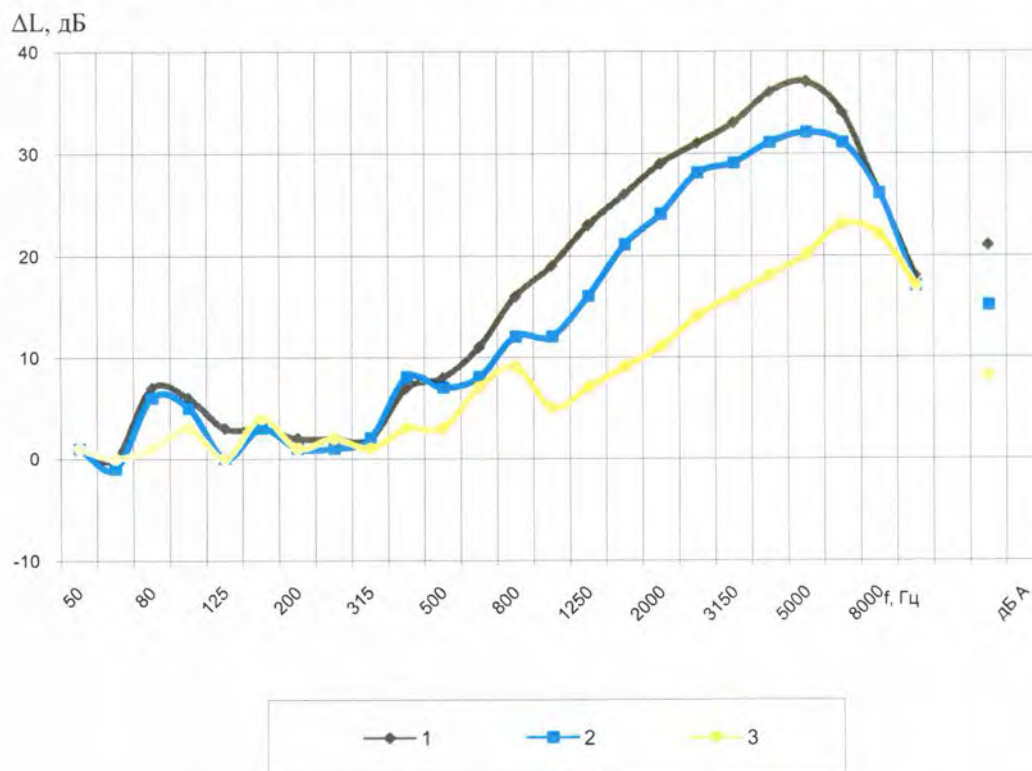
1 – покрытие TecsoundFT75; 2 – покрытие TecsoundFT 55 PP; 3 – покрытие SYAl Рисунок 3.2 – Эффективность покрытий на трубе диаметром 200 мм
